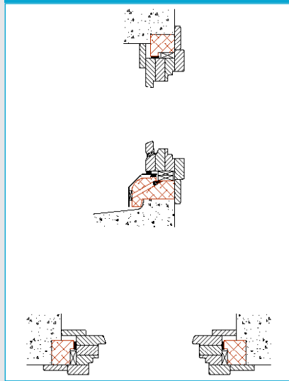
Ailette rénovation de 17 mm en base (option couvre-joints, bavette alu)
