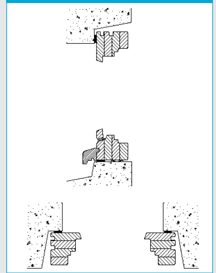
Dormant de 80 mm avec pièce d'appui (option couvre-joints)
