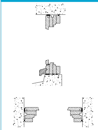
Dormant de 80 mm avec pièce d'appui (option couvre-joints)
